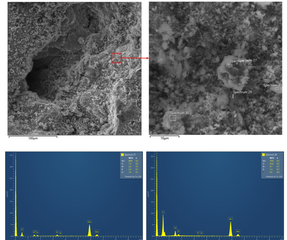
štruktúra Mn rudy Gabun po redukcii pri 600 °C v atmosfére H 2 (čas redukcie - 30 min.)
