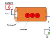
Obr. 80 Aparatúra pre redukciu peliet v 100 % atmosfére vodíka, zariadenie LAC
